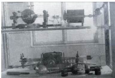
Fig. nr. 10 – Colecția de tuburi Röntgen cu gaz (catod rece) cu răcire prin aripioare regeneratoare cu scânteie
